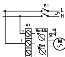
Schemat elektryczny 4
