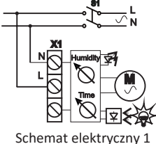
Schemat elektryczny 1
